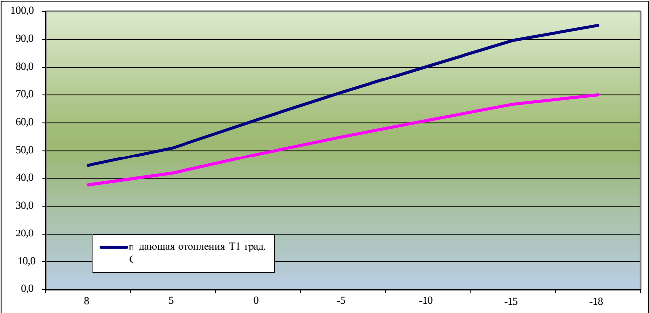
Температурный гра ик центрального качественного регулирования
